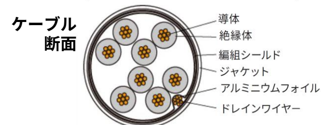
STP 構造図 (2重シールド)
