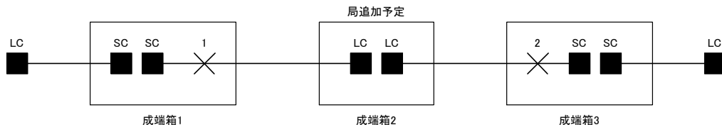
図 4.1.2-2 接続例
